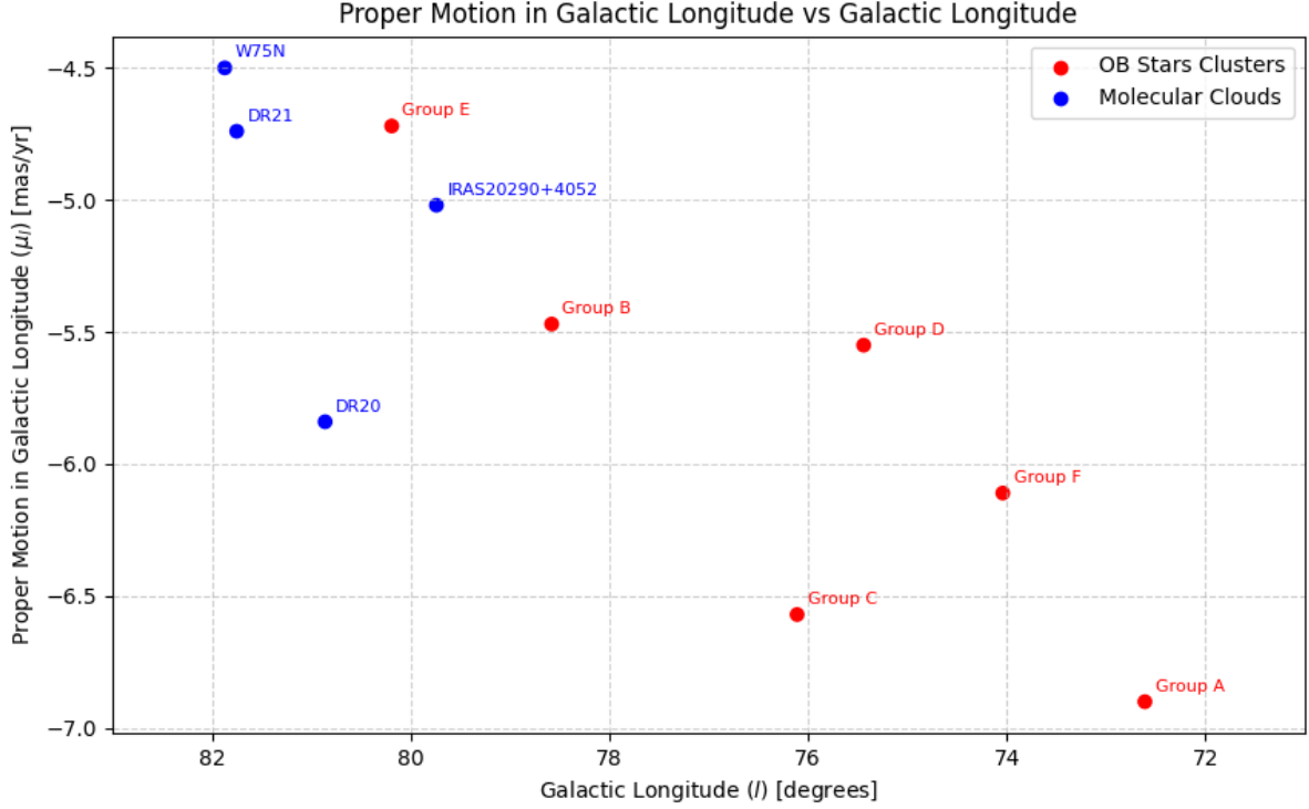
FIGURE 7 – Mouvement propre selon la longitude galactique \mu_l en fonction de la longitude galactique l , les nuages moléculaires sont en bleus et les amas d'étoiles OB en rouge
