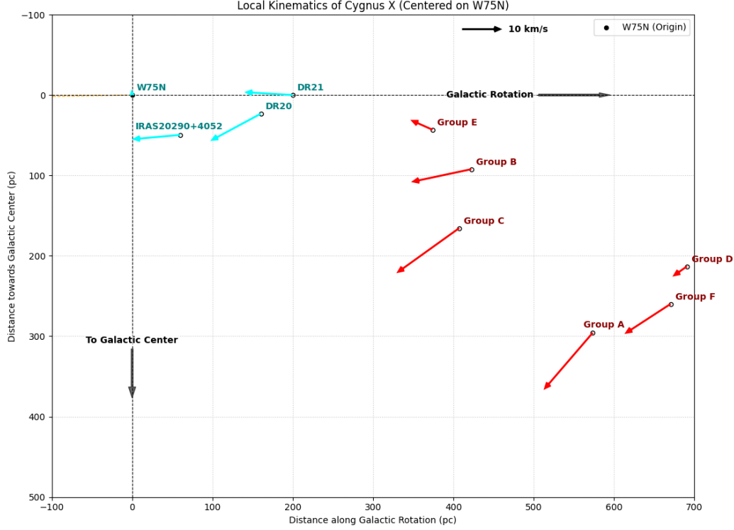
FIGURE 8 – Projection des vitesses U_{pec} et V_{pec} des nuages moléculaires et des groupes d'étoiles massives sur le plan galactique. Le graphique est centré sur le nuage W75N. L'abscisse est la distance selon la rotation de la galaxie et l'ordonnée est la distance vers le centre galactique. La ligne jaune indique la direction du Soleil. Les nuages moléculaires sont en cyan et les groupes d'étoiles en rouge.
